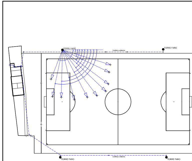
PIANTA CAMPO SPORTIVO CON PUNTAMENTI TORRI FARO
