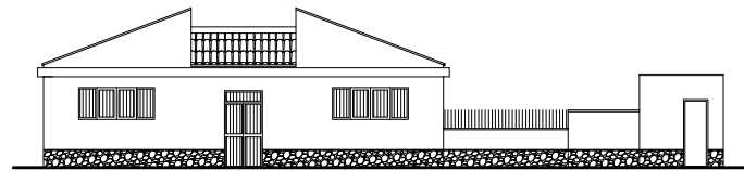
PROSPETTO EST
