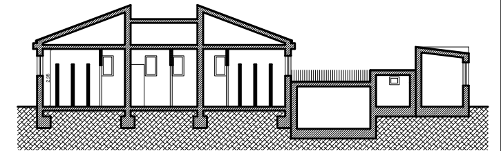
SEZIONE A-A
