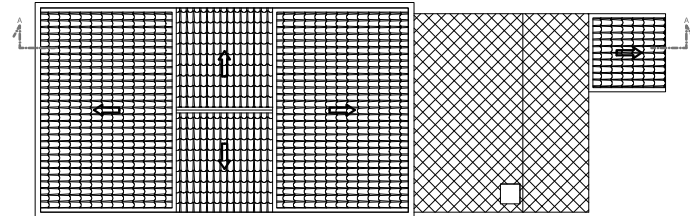
PIANTA COPERTURA
